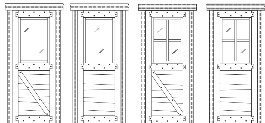
cod. T-23 cod. T-13 cod. T-25 cod. T-15
