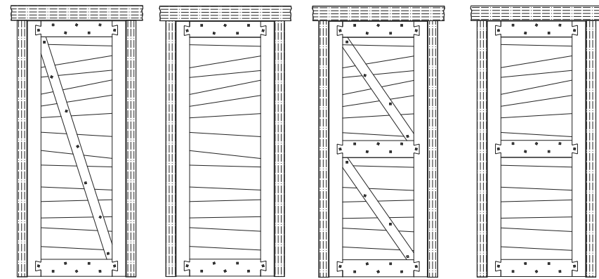
cod. T-21 cod. T-11 cod. T-24 cod. T-14
